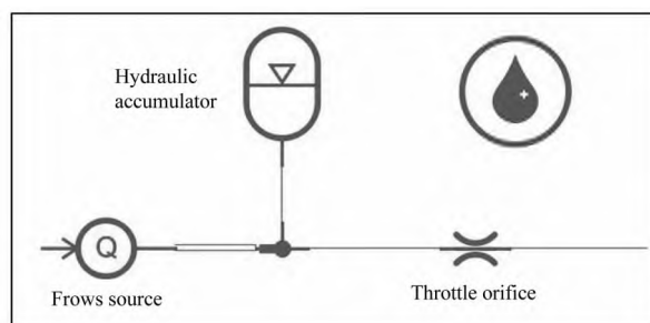
图5 液压阻容滤波结构
