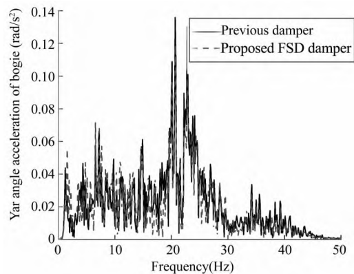
(b) 构架摇头频谱分析
