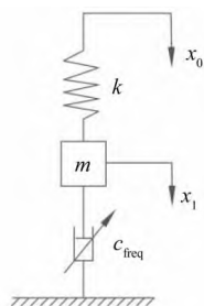
图7 FSD 简化模型
