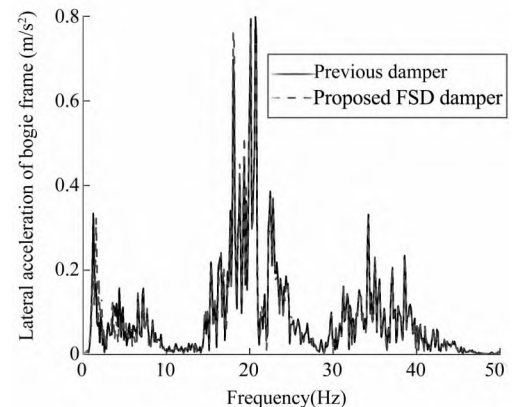
(a) 构架横移频谱分析
