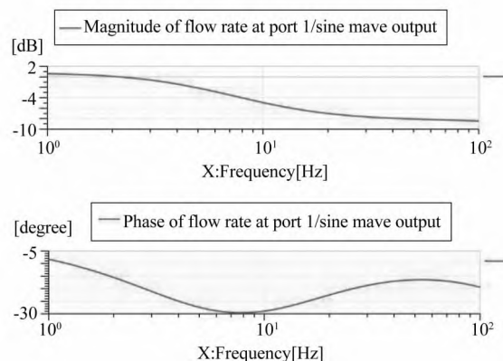
图6 液压阻容滤波结构频谱分析图
